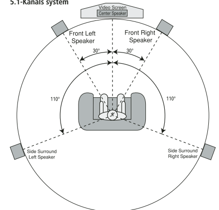
A. Uppställning av högtalare för främre kanaler med vanlig TV-apparat eller bakprojektorbildskärm
